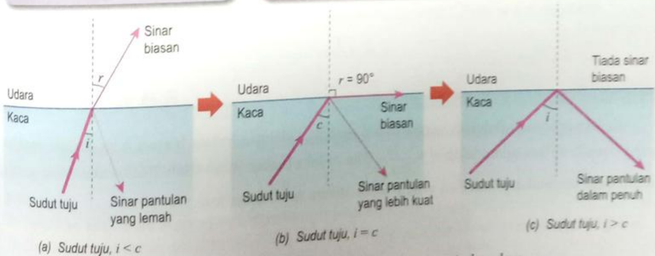
Rajah 6.19 Perambatan sinar cahaya dari kaca menuju ke udara
