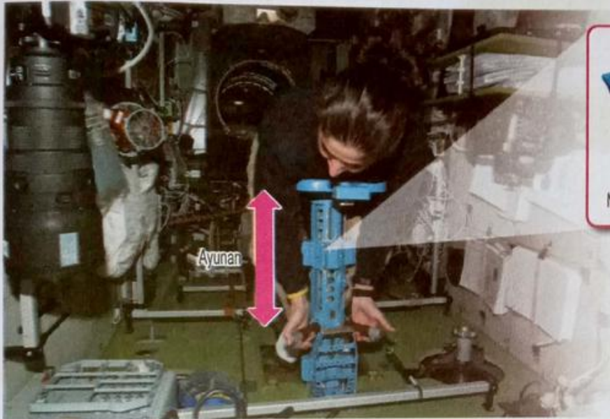
Gambar foto 2.6 Penggunaan neraca inersia oleh angkasawan
