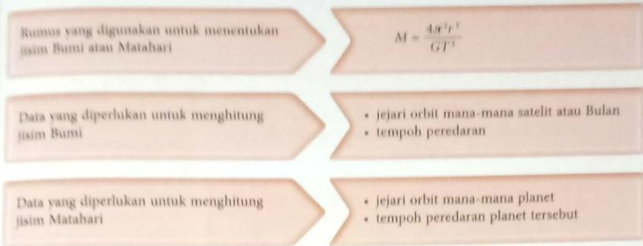
Rajah 3.22 Rumus dan data yang digunakan untuk menghitung jisim Bumi dan Matahari
